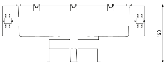
Gesamthöhe mit Schalungsring
